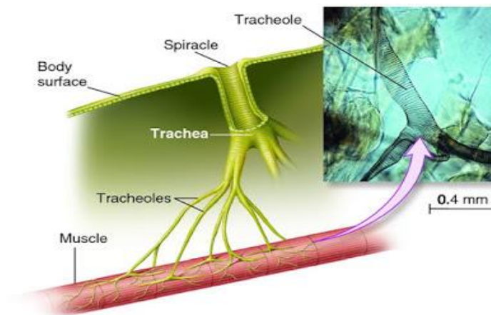
Gambar 7. Struktur sistem pernapasan serangga Sumber: (Jasin, 1983).
