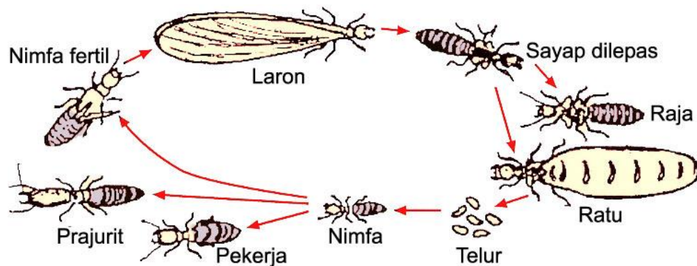
Gambar 2. Siklus hidup rayap Sumber : Nandika, dkk 2003
