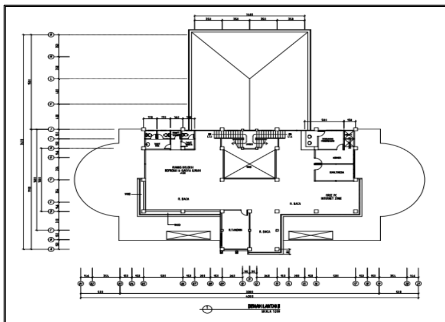
Gambar 3.6: Denah Lantai III (Ketiga)
