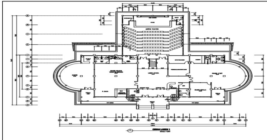
Gambar 3.2 Denah Lantai II (Kedua)
