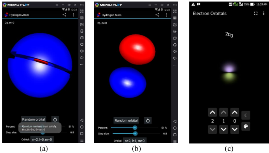
Gambar 3. Visualisasi: (a) orbital 2s, (b) orbital 2p menggunakan aplikasi Hydrogen Atom ; dan (c) orbital 2p menggunakan aplikasi Electron Orbitals .
