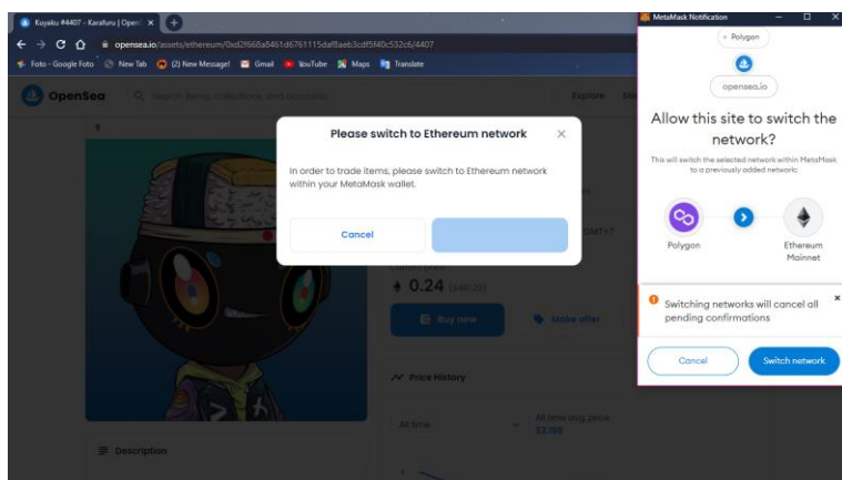
GAMBAR 3. 13 PEMBELIAN NFT
