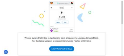
GAMBAR 3. 2 MENGUNDUH METAMASK
