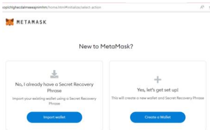
GAMBAR 3. 5 VERTIFIKASI METAMASK
