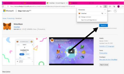
GAMBAR 3. 3 MASUK METAMASK
