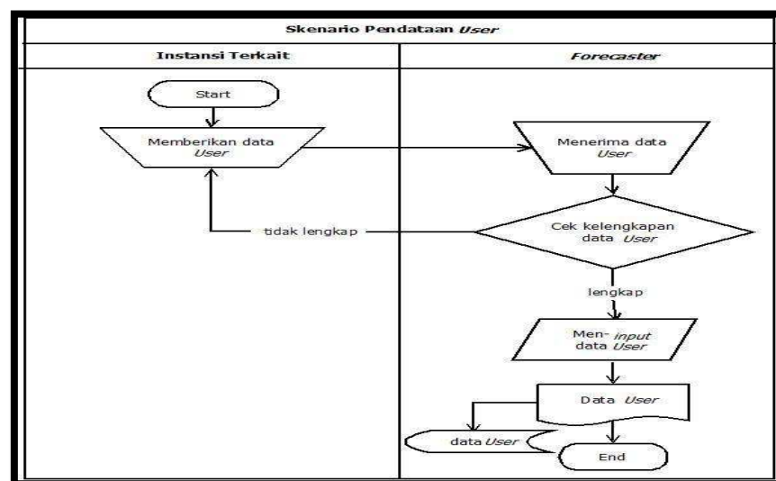
Gambar 3.2 Skenario pendataan user yang sedang berjalan
