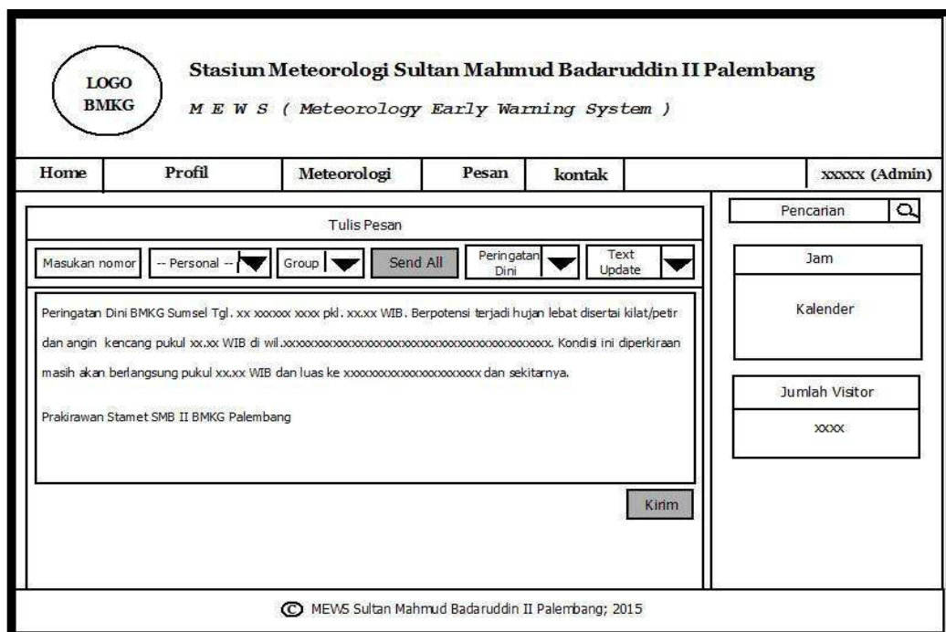
Gambar 3.29 Rancangan interface tulis pesan prakiraan.
